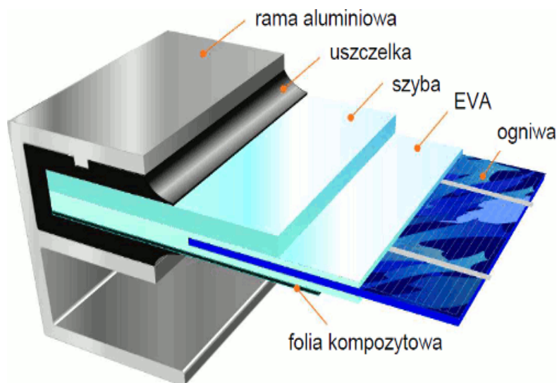
Rys nr 4. Budowa jednostki wytwórczej farmy fotowoltaicznej
