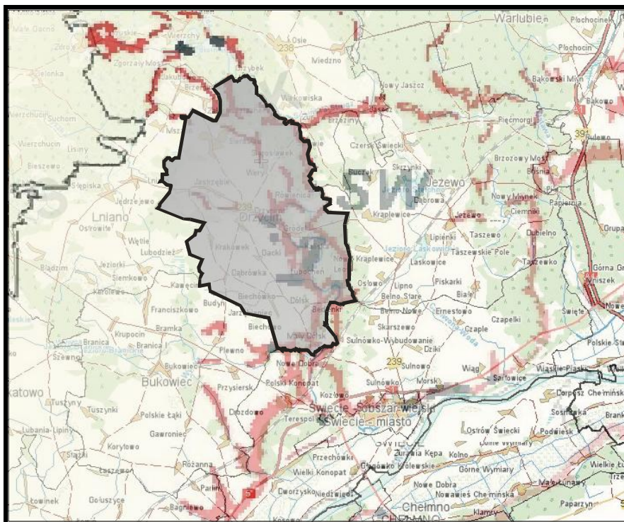
Rysunek 15. Tereny predysponowane do występowania ruchów masowych (kolor czerwony), czarną linią zaznaczono granice gminy, wg PIG.
